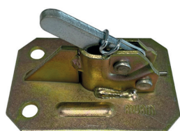
Tensor grapa metálica
