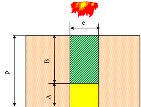
- Sección Transversal Tipo 1-
