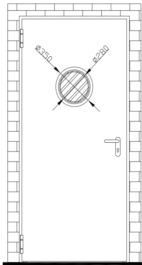
VIDRIO MULTIUSO EN PUERTAS DE 53 mm
